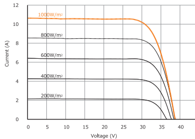
放射照度別 I-V カーブ
