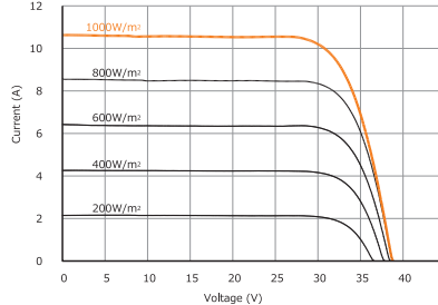
放射照度別 I-V カーブ
